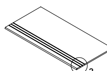
step tread grooved nez de marche creusé stufenplatte mit rillen degrau sulcado 30x60 NR . ASR MP-6240 A MP-6270 30x90 NR . ASR MP-6430
